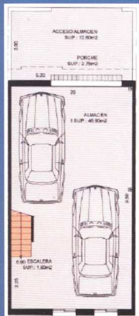
semisótano
