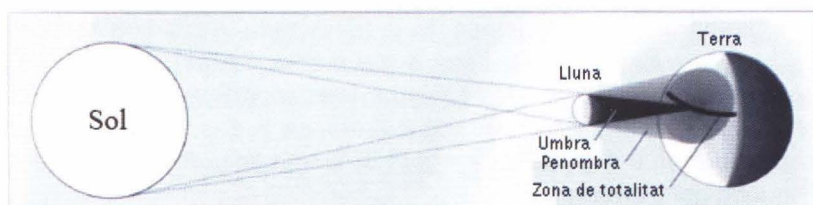
Esquema d'un eclipsi total: l'ombra de la Lluna arriba a la Terra
