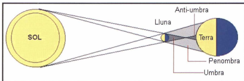
Esquema d'un eclipsi anular: l'ombra de la Lluna no arriba a la Terra
