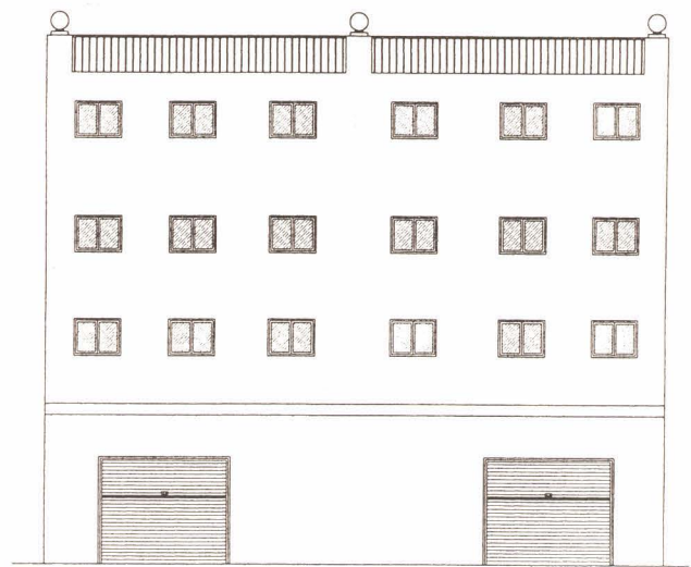
Alzado C/ Santa Catalina
