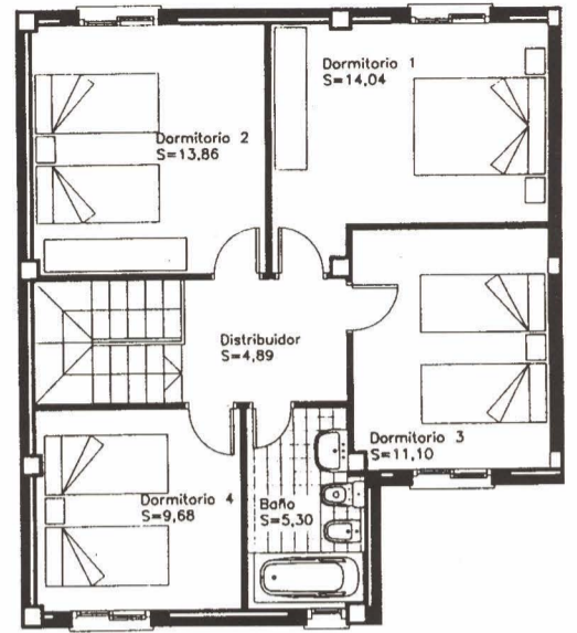
PLANTA PRIMERA Superficie construida por vivienda 73,36 m2.
