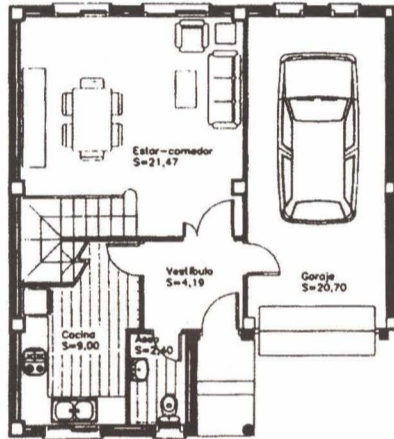
PLANTA BAJA Superficie construida por vivienda 70,21 m 2 .
