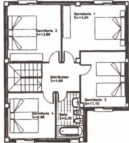
PLANTA PRIMERA Superficie construida por vivienda 73,36 m 2 .
