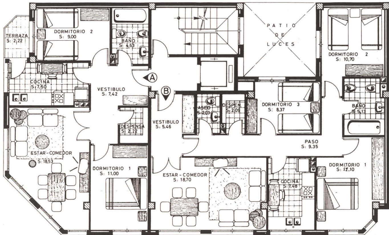
PLANTA DISTRIBUCION.
