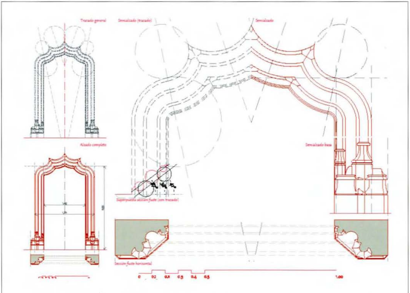
Fig. 8: Lámina de presentación de la Portada 5 (Dór 5): alzado, sección horizontal y trazados de jamba y arco. Fuente: Propia
