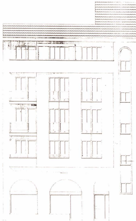
ALZADO
