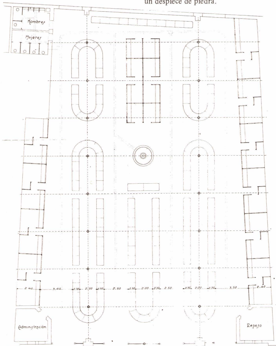
ESCALA DE 1:100
