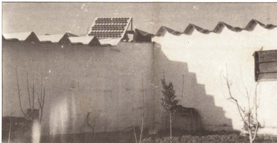
INSTALACION DE TRES PANELES EN UNA GRANJA DE CONEJOS
