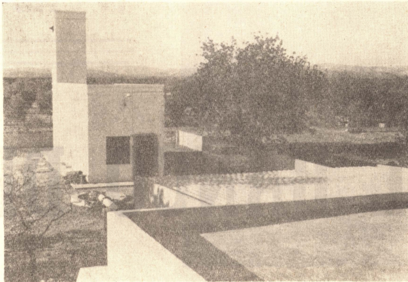
Pozo de Ntra. Sra. de la Misericordia: instalación del transformador y balsas
