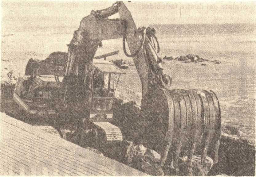
Obras de reconstrucción del muro del Paseo de Colón, destruido por los temporales.
