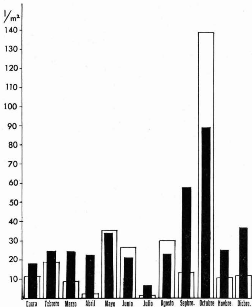
FIG. 4. — Valores mensuales de la lluvia recogida, expresados en litros por metro cuadrado. Los rectángulos en negro representan los valores medios de los últimos diecisiete años.
