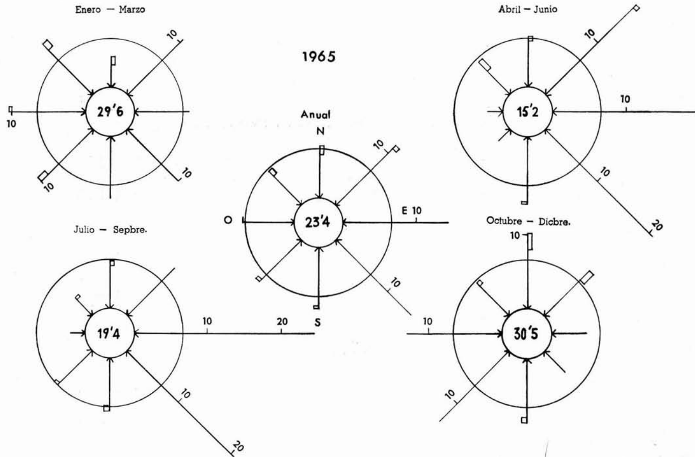
FIG. 3.— Vientos: tanto por ciento de frecuencias e intensidad en los cuatro trimestres del año y resumen anual. En el centro de cada figura se indica el porcentaje de calmas. Al lado derecho de las flechas, cuando es posible, se marca una escala de porcentajes para los vientos débiles y fuertes. Los rectángulos al lado izquierdo de las flechas representan, en el sentido longitudinal, la frecuencia de los vientos fuertes cuando existen.
