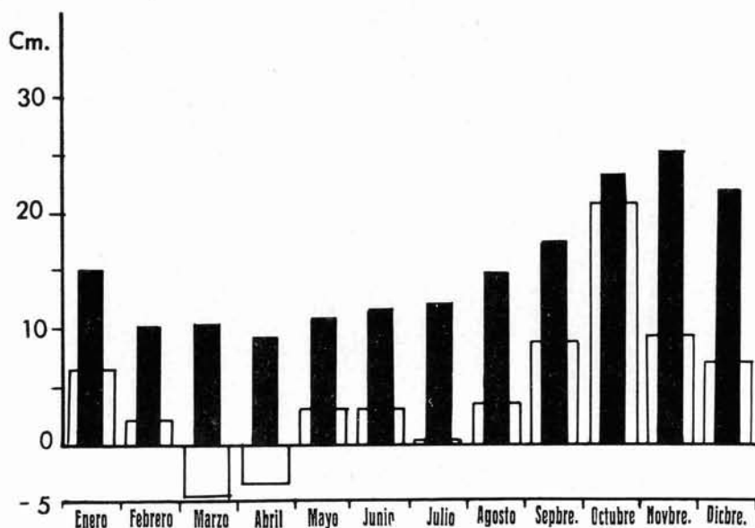
FIG. 5. — Valores medios mensuales del nivel del agua del mar en el puerto. Los rectángulos en negro representan los valores medios de los últimos trece años.
