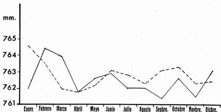
FIG. 2. — Valores medios mensuales de la presión atmosférica a 0°C y al nivel del mar. La línea de trazos representa el valor medio durante los últimos diecisiete años.
