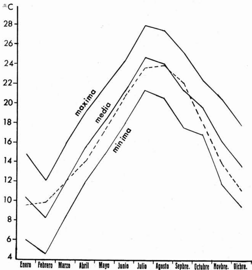
FIG. 1. — Valores medios mensuales de las temperaturas máximas, medias y mínimas. La línea de puntos representa el valor medio durante los últimos diecisiete años.
