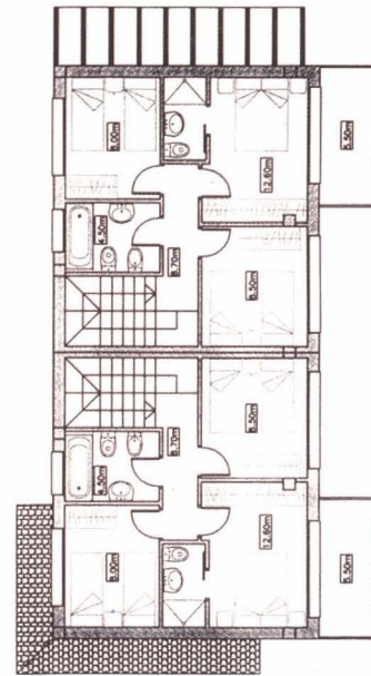
PLANTA PRIMERA
