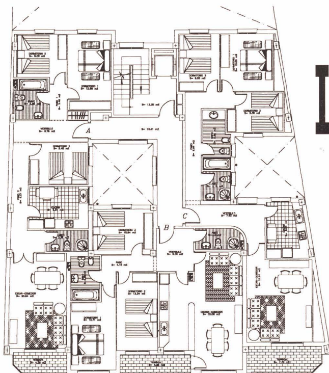
PLANTA PISOS DISTRIBUCION
