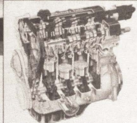
Cuatro cilindros en bloque de aluminio. 100CV. de potencia a 6.000 rpm.
