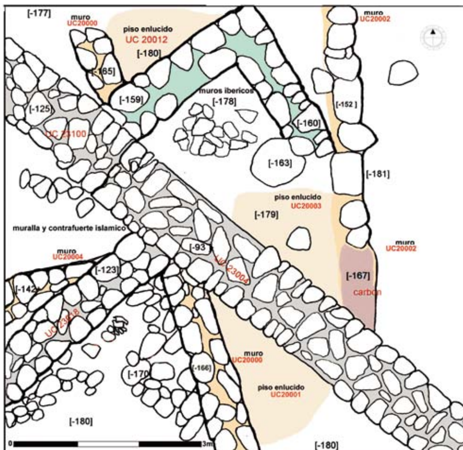
Figura 10.- Planimetría de estructuras de la Fase II en el sector Q-20.
